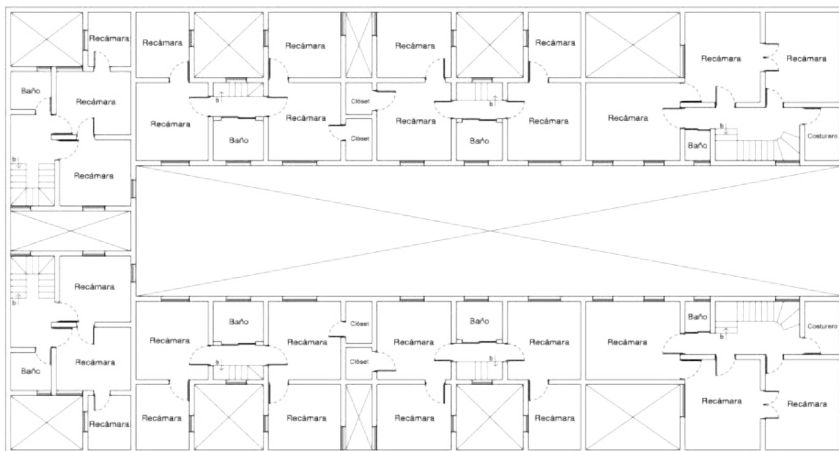
Dibujo: César Ivan Cuevas y Bruno Langle Tamayo, a partir del levantamiento publicado en: Vicente Martín Hernández, Arquitectura doméstica de la Ciudad de México 1890-1925 (México, UNAM, 1981, pp. 141 y 142).
