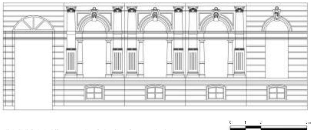
Dibujo de la fachada de la casona en la calle de Jalapa núm. 13, en la colonia Roma. Elaboración: Jonathan Manuel Herrera Sagundo, julio de 2013.
